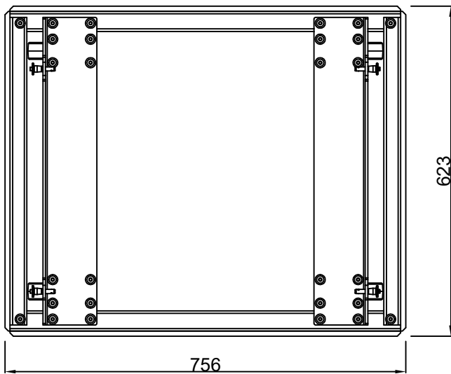
上面図
