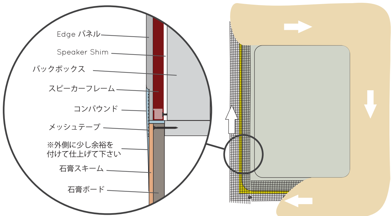
施工詳細 - ウェットスキームによる補強
